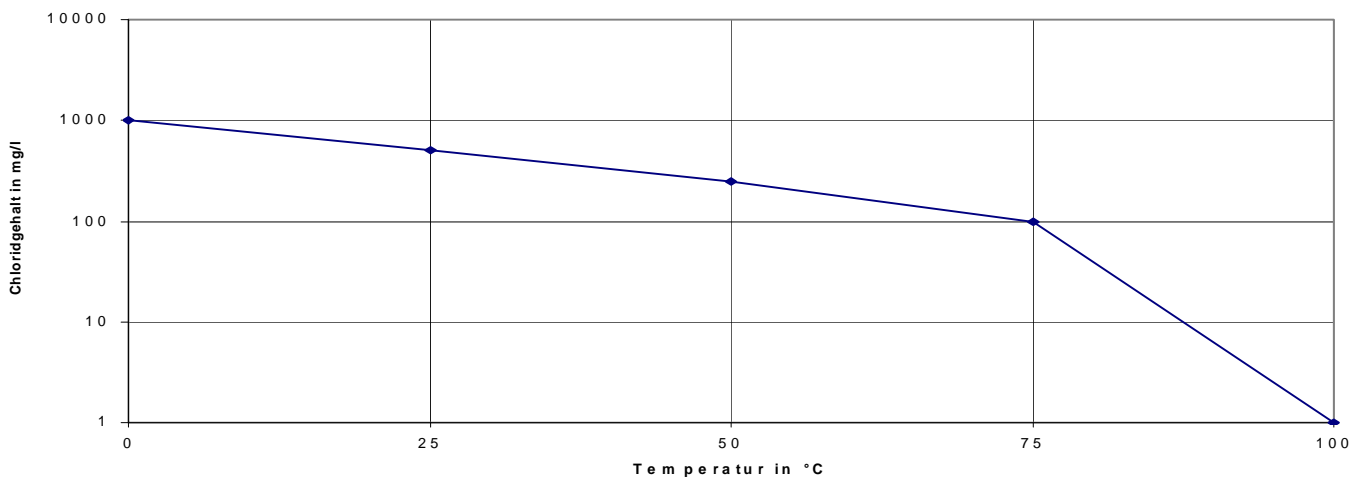
zulässiger Chloridionengehalt in Abhängigkeit von der Temperatur
